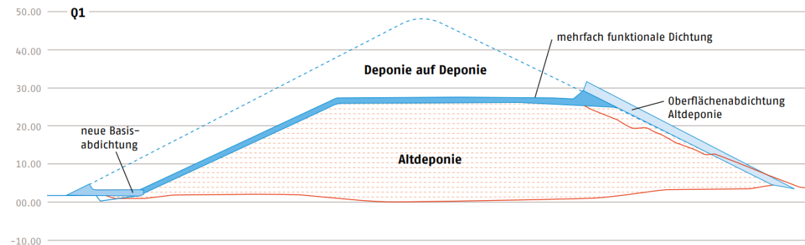
Abb. 4.2: Beispiel Kombination aus vorgelagerter Erweiterung „Deponie overlapped“ und „Deponie on top“ (BIENER et al. 2011)
